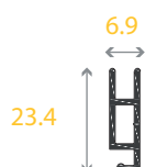
2331 Marco Malla
