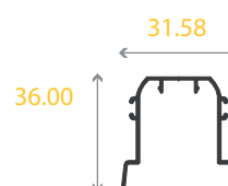
3427 Doble Entrecierre
