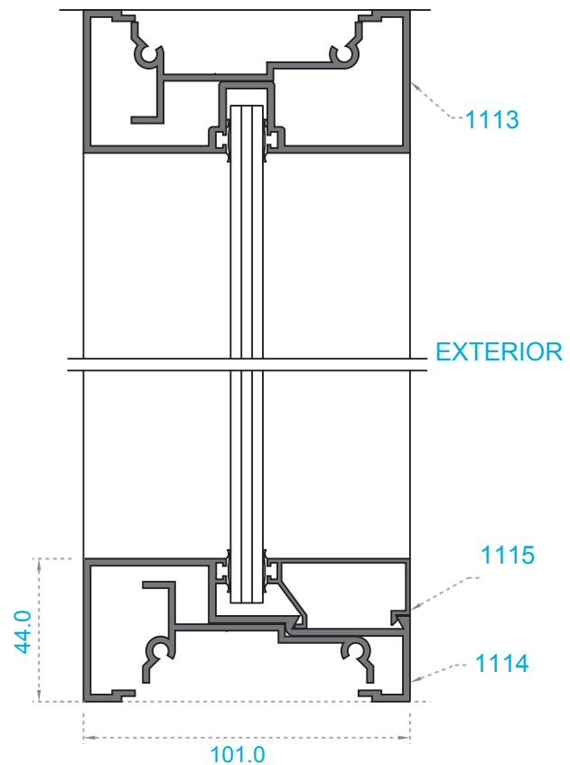
SECCIÓN HORIZONTAL (B - B)
